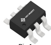
Pin 1 SOT-363 (SC-70-6)
