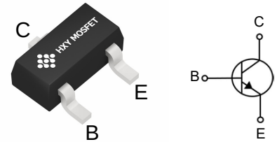
SOT-23
