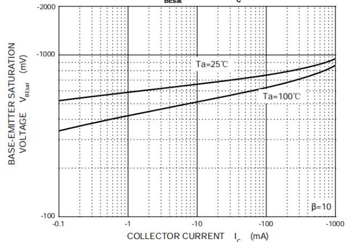
V_{BEsat} — I_c
