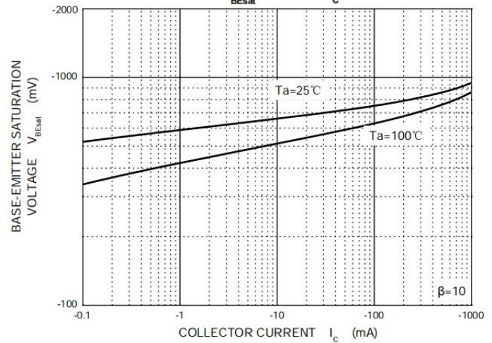
V_{BEsat} — I_c
