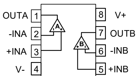
TSSOP-8
