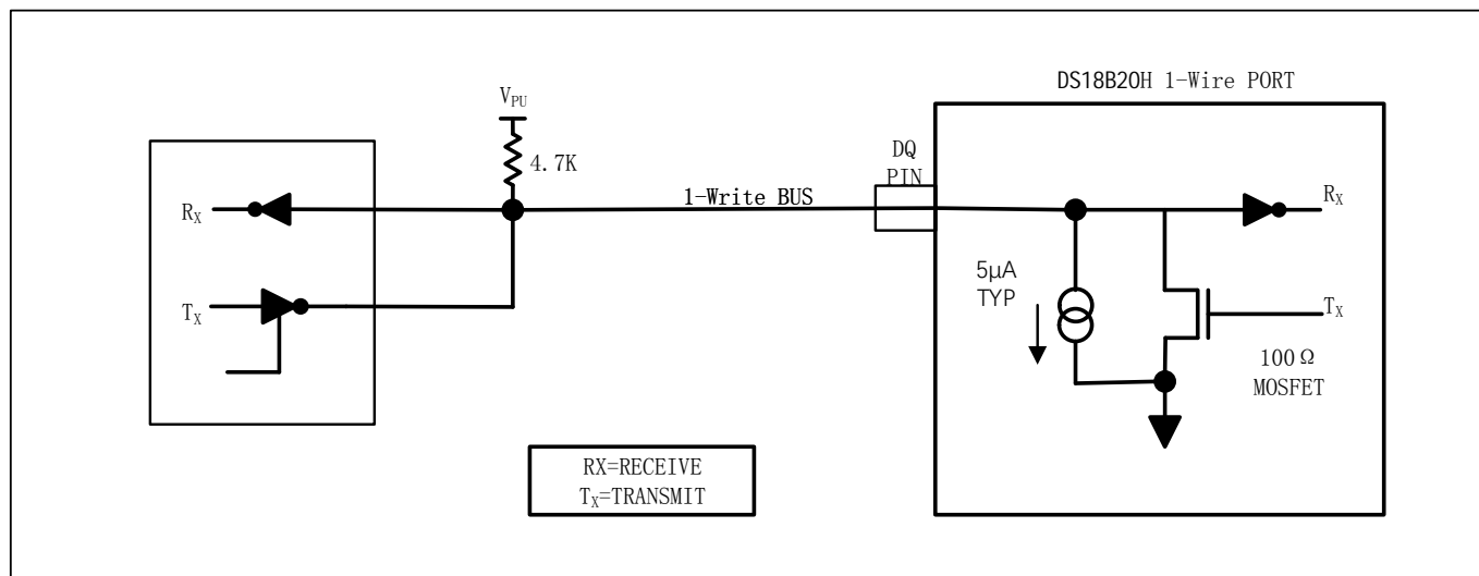
图 10. 硬件结构图
