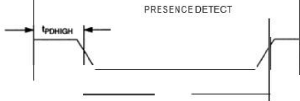
图 18. 时序
