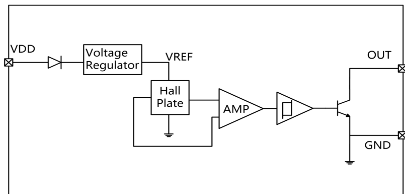
SS41F 功能框图
