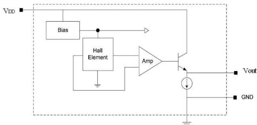
AH602 功能框图
