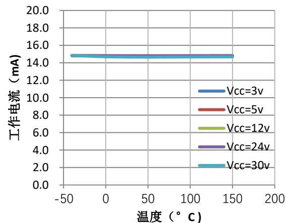
V_{CC}=3.0\sim30V , 平均电源电流 (低) 输出特性曲线
