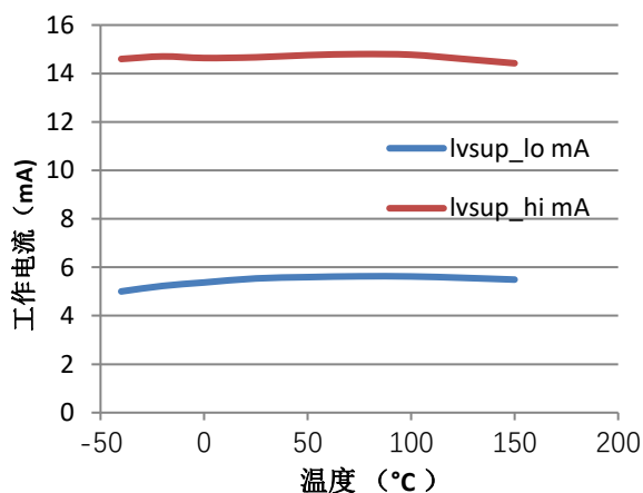
V_{CC}=3.0\sim30V , 平均电源电流 (低) 输出特性曲线
