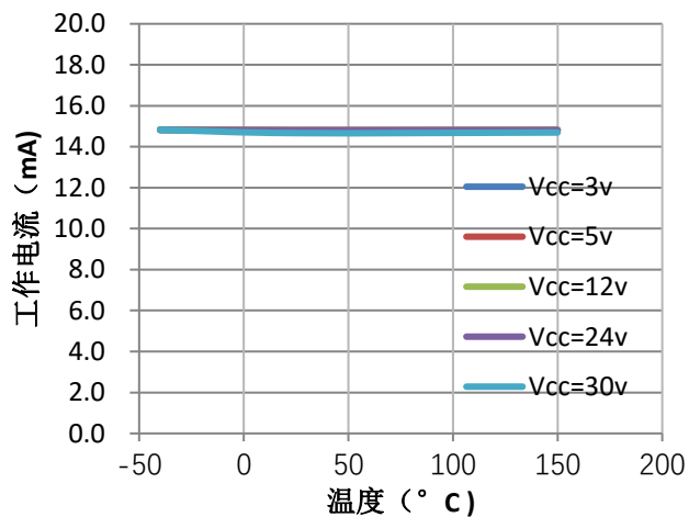
V_{CC}=3.0\sim30V , 平均电源电流 (低) 输出特性曲线
