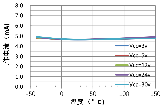
V_{CC}=3.0\sim30V , 平均电源电流 (低) 输出特性曲线
