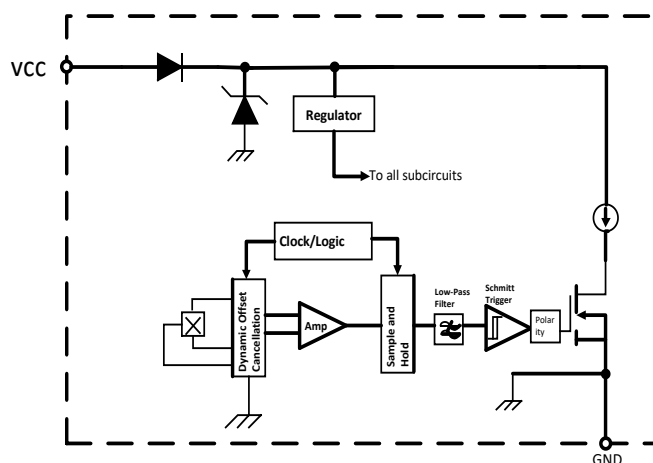
AH542 功能框图
