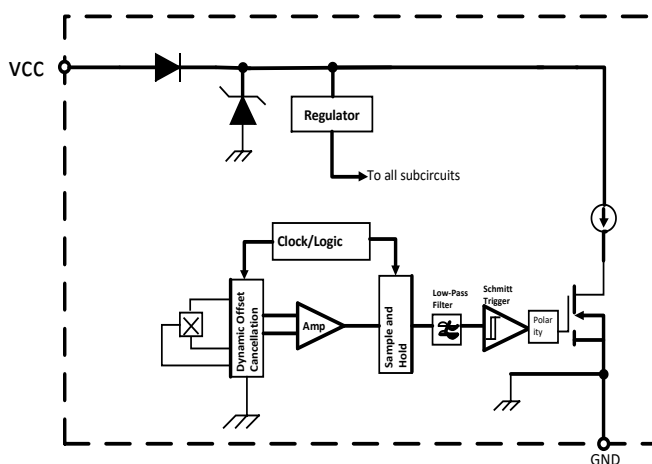
AH541 功能框图
