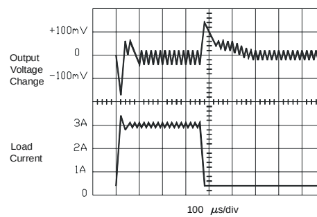
负载瞬态响应
