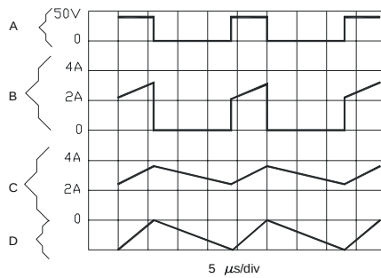
开关波形
