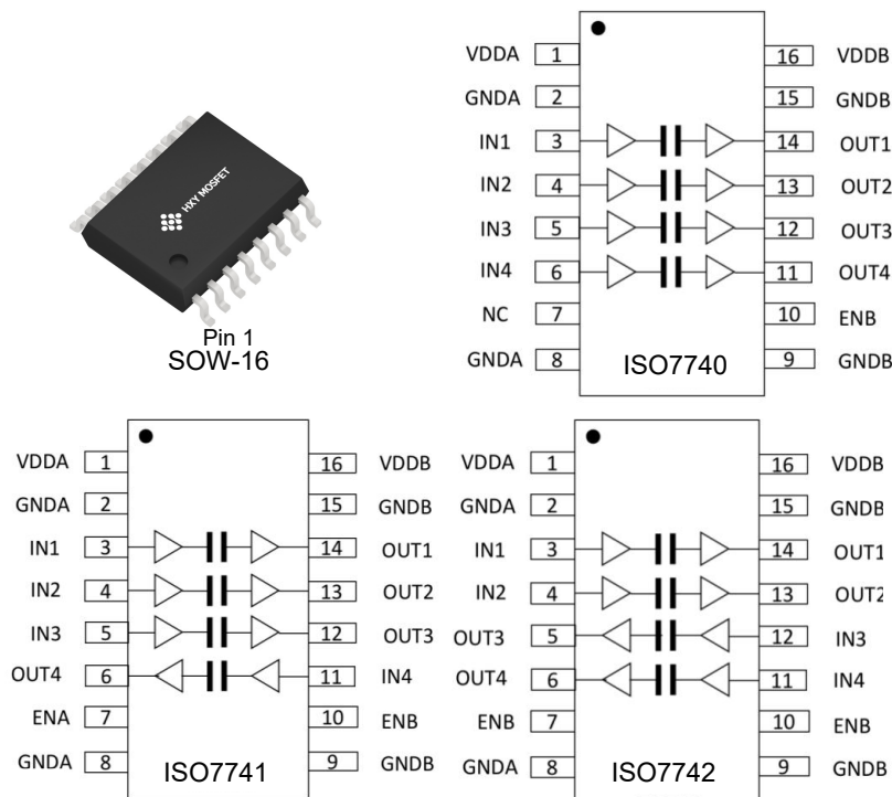
图 2-1 ISO774x顶部视图表
