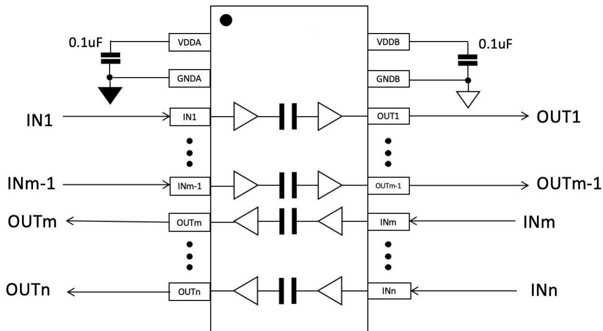
图 6-1 ISO774x系列数字隔离器应用原理图
