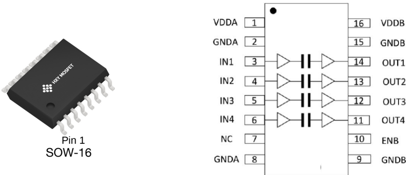
图 2-1 CEU8740U1W顶部视图
