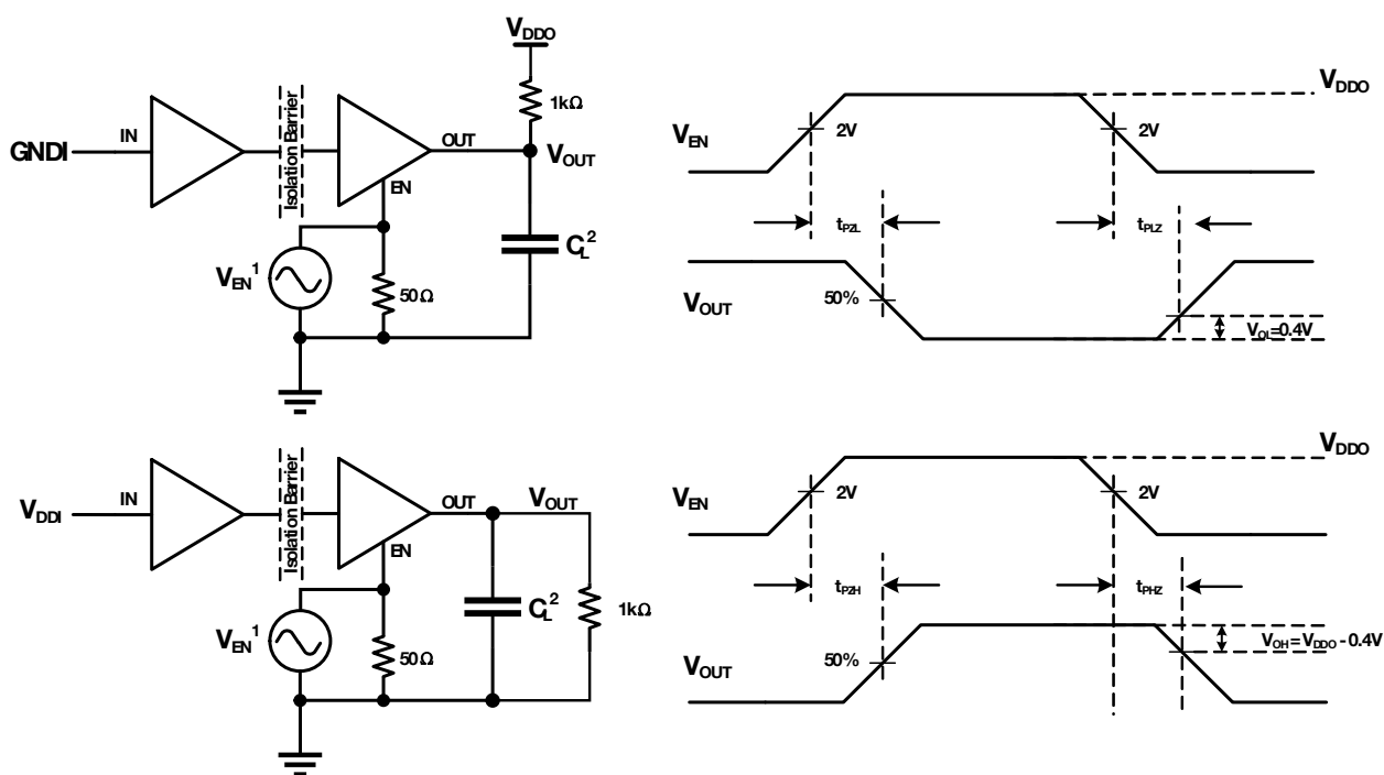
图 4-1时序特性测试电路和电压波形
