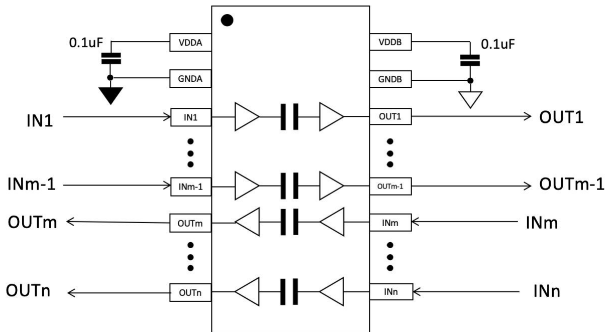
图 6-1 CEU8740U1W系列数字隔离器应用原理图
