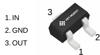
SOT-523
