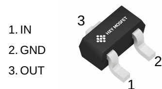
SOT-523 (SC-75)
