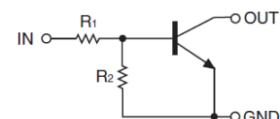
SOT-523 (SC-75)
