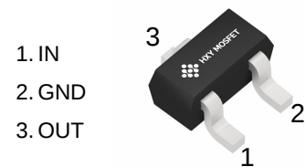
SOT-523 (SOT-416)
