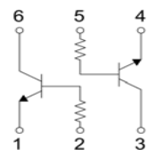
SOT-363
