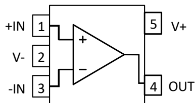
SOT-353(SC70-5)
