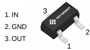
SOT-23
