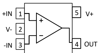
SOT-23-5L
