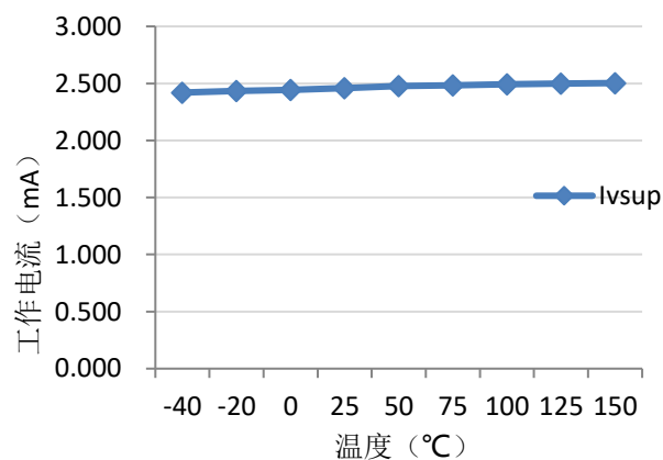
V_{CC}=5V , 芯片工作电源电流随温度变化特性曲线
