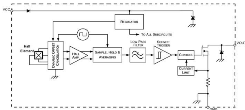
AH512 功能框图
