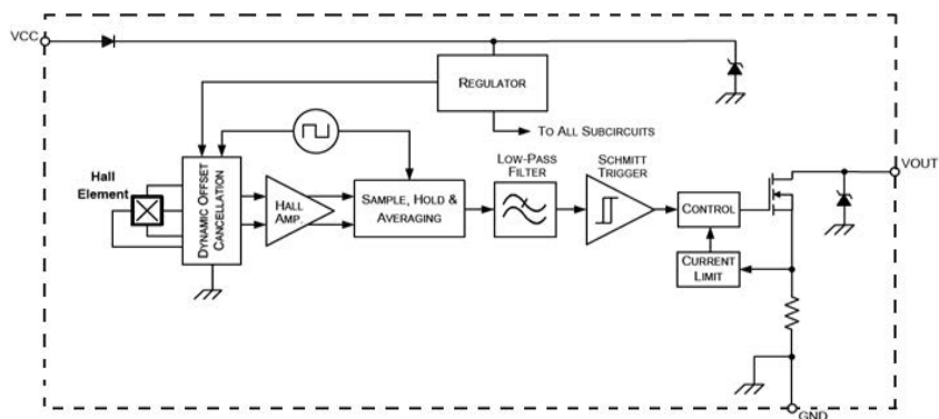
AH502 功能框图
