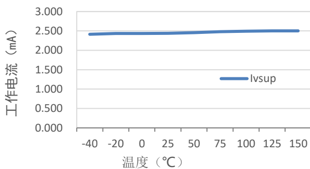
V_{CC}=5V , 芯片工作电源电流随温度变化特性曲线
