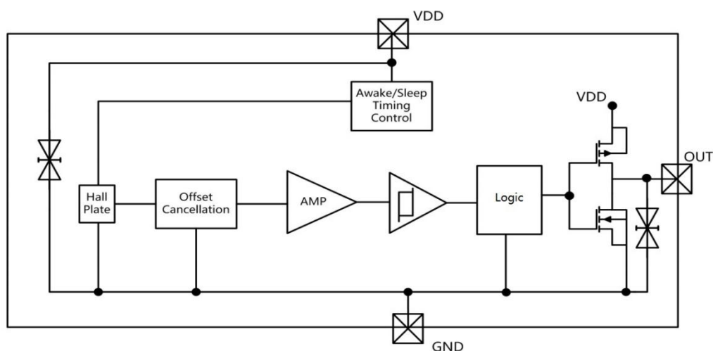
AH469 功能框图
