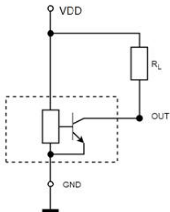
典型应用电路例1
