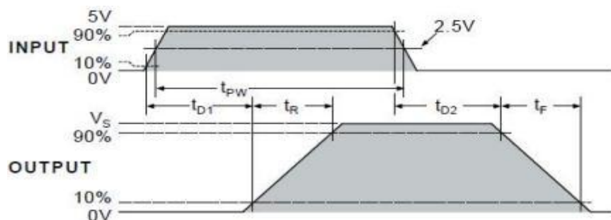
输入输出（B通道同相）波形图
