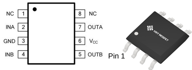
SOP-8(SOIC-8) 顶视图
