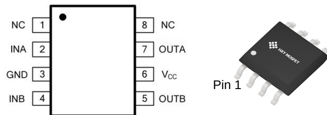
SOP-8(SOIC-8)顶视图
