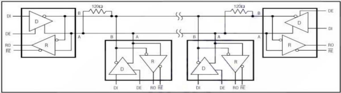
典型应用图
