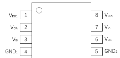
图 2. 管脚定义
