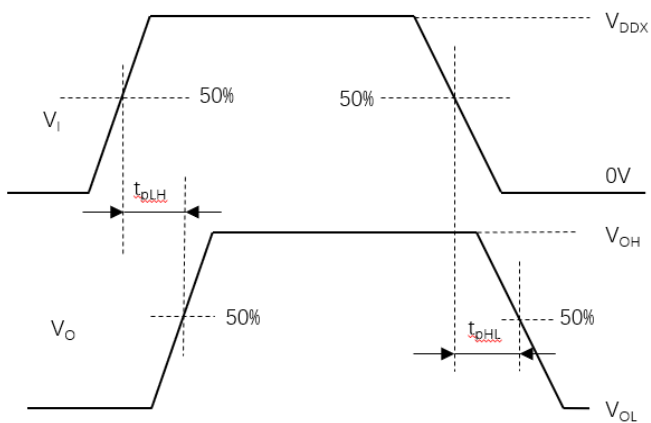
图 8 . 传输延迟时间波形测量
