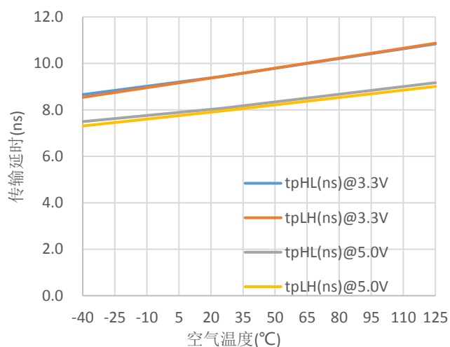
图 6 . 传输延时 vs. 空气温度
