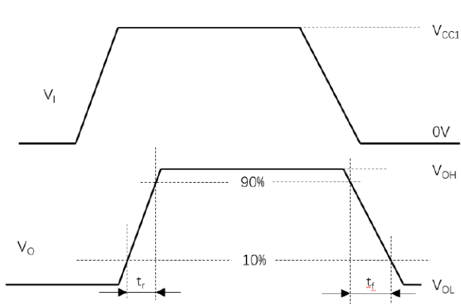
图 7 . 传输时间波形测量
