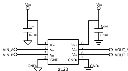
图 2. 应用简图
