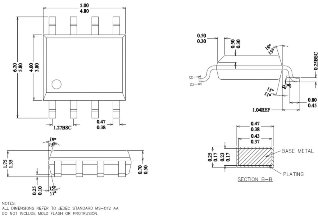
图 12. SOP-8 封装外形尺寸-尺寸单位(mm)
