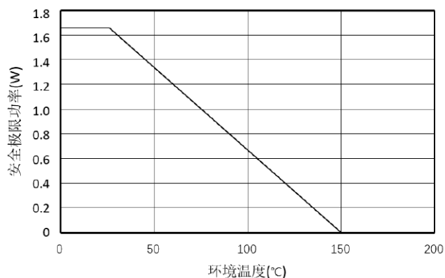
图 4.热降额曲线，依据 DIN V VDE V 0884-10 的安全限值与环境温度的关系
