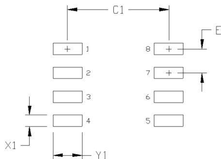
图 20.8 引脚SOP 封装焊盘图案
