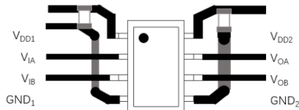
图 9 .推荐的印刷电路板布局
