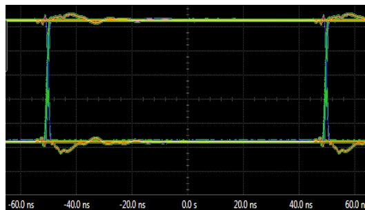
图 10.眼图
