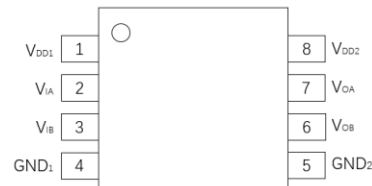
图 3. 管脚定义
