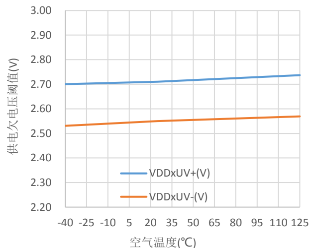
图 5.UVLO vs. 空气温度
