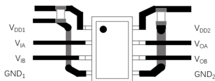
图 9 .推荐的印刷电路板布局
