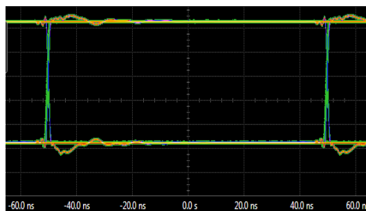
图 10.眼图
