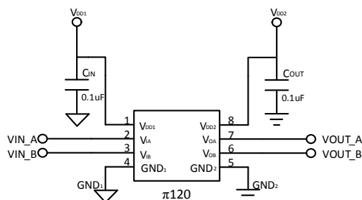
图 2. 应用简图
