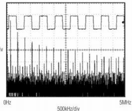
图7：发送150KHz信号时的驱动器输出波形
