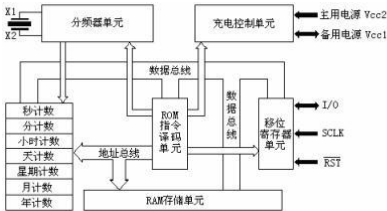
图 1 DS1302ZN+T&R 内部框图
