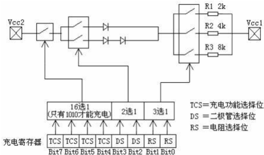
图 4 DS1302ZN+T&R 可编程慢速充电器
