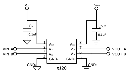
图 2. 应用简图
