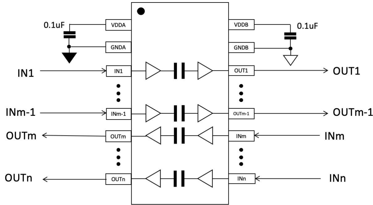
图 6-1 SOW-16 CEU872x典型应用电路
