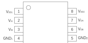
图 3. 管脚定义
