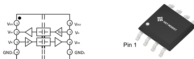
图 1. 功能框图
