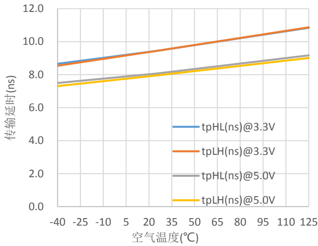
图 5 . 传输延时 vs. 空气温度
