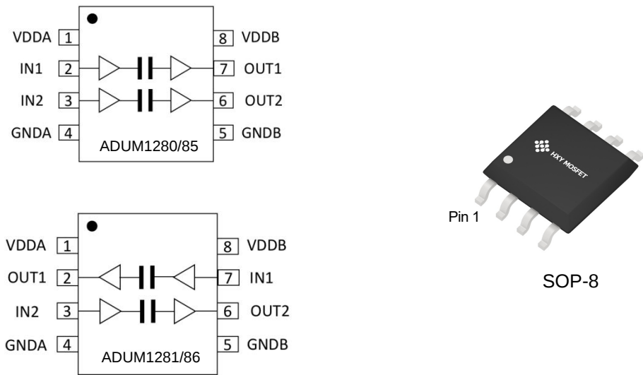
图 2-1 ADUM128x SOP-8 封装顶部视图
