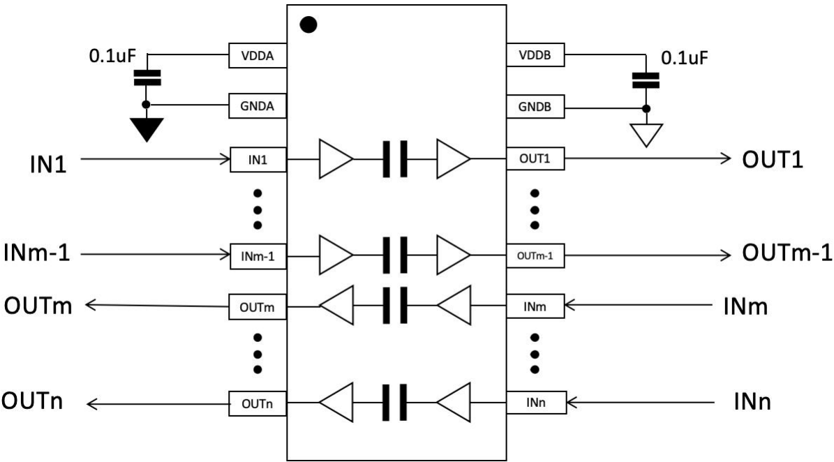
图 6-1 SOW-16 ADUM128x 典型应用电路
