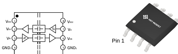
图 1. 功能框图
