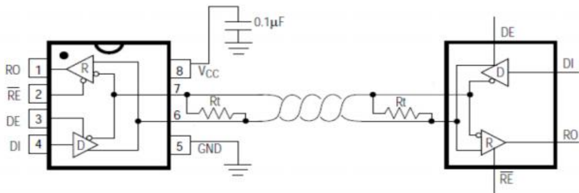
图 1：MAX485ESA典型半双工应用电路
