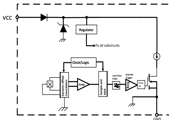
HXY543 功能框图
