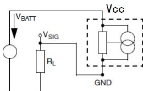
典型应用电路（1）
