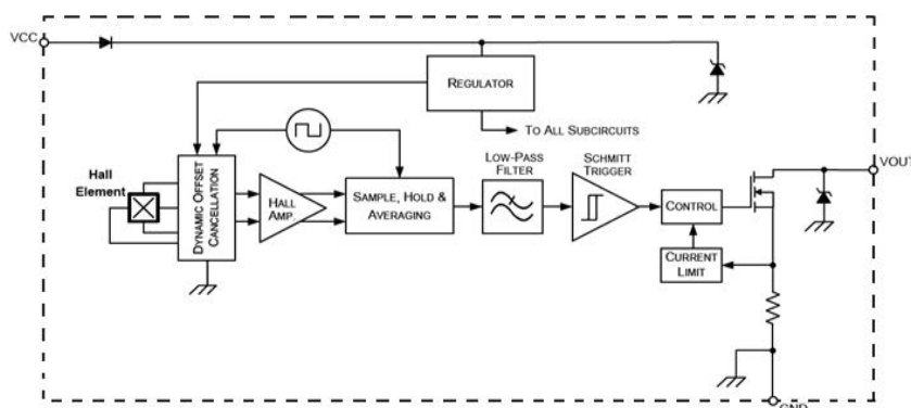
HXY510 功能框图
