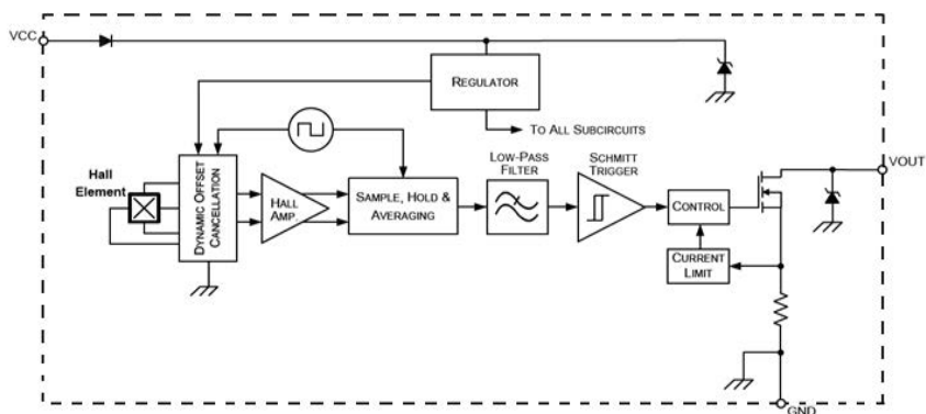
HXY509 功能框图
