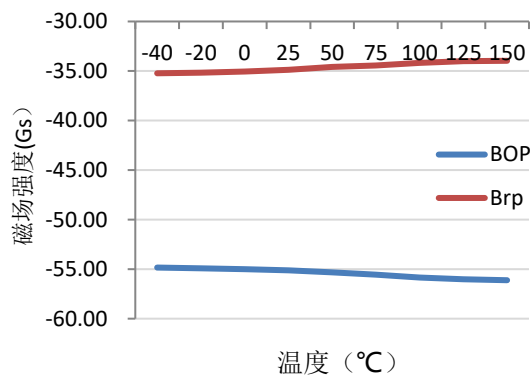
V_{CC}=5V , 芯片工作点与释放点温度变化特性曲线
