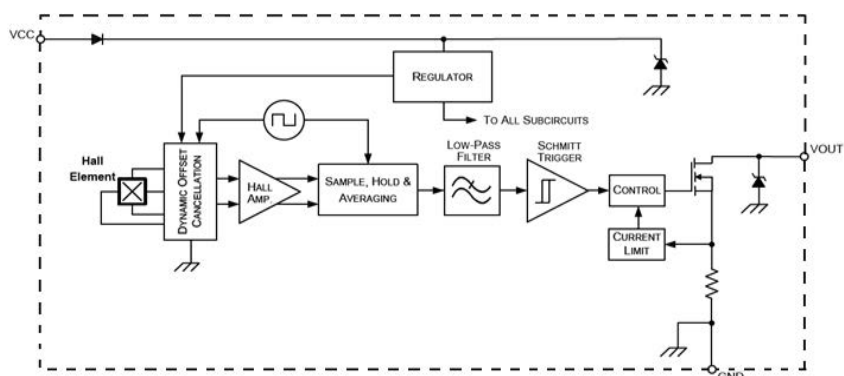
HXY506 功能框图
