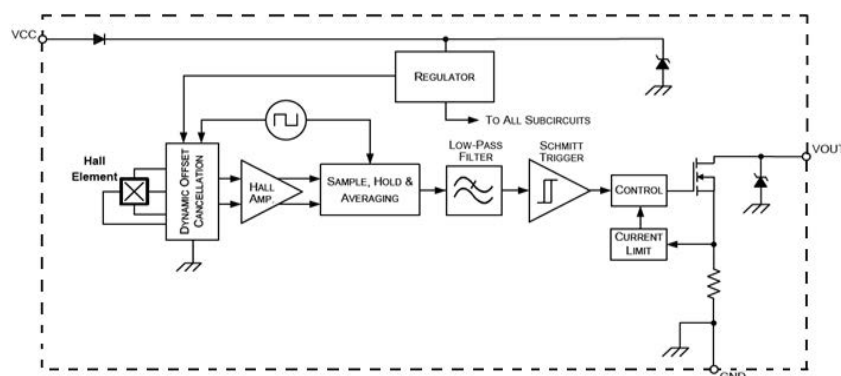
HXY505 功能框图
