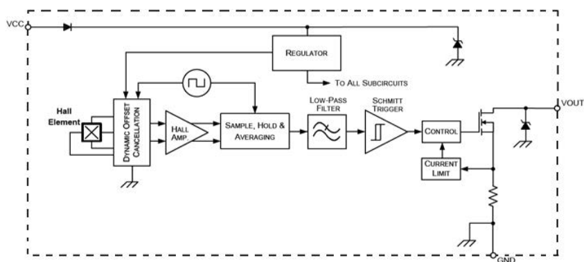
HXY503功能框图
