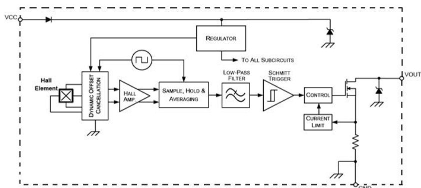
HXY502功能框图
