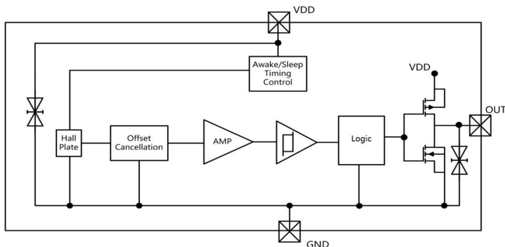
HXY466 功能框图
