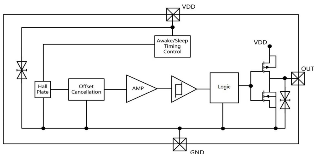
HXY462 功能框图
